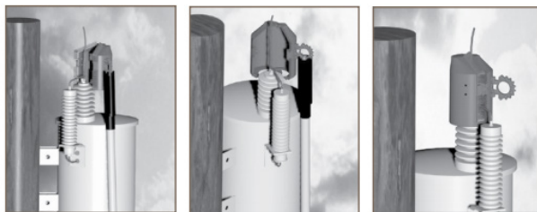
Mit dem «Hot Stick» ist eine Montage unter Spannung möglich
