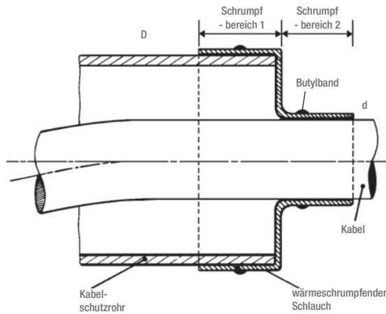
KABELSCHUTZROHRABDICHTUNGEN CADS
